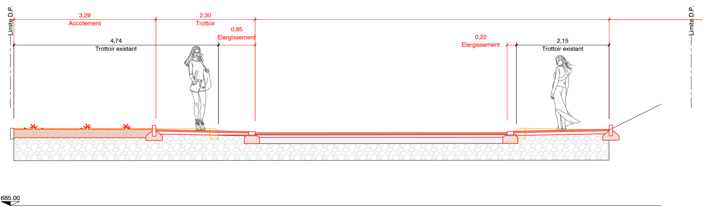
Coupe B-B: 1:50
